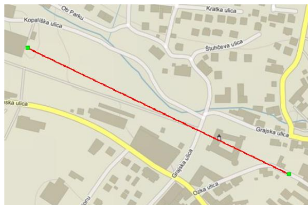
Slika 17: Profil površja med OŠ Pohorskega odreda in Ozko ulico (vir: PISO)
