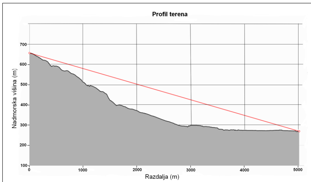
Slika 20: Profil površja območja Slovenske Bistrice med vrhom Borje in JV obmestnim predelom (označeno na sliki 19)
