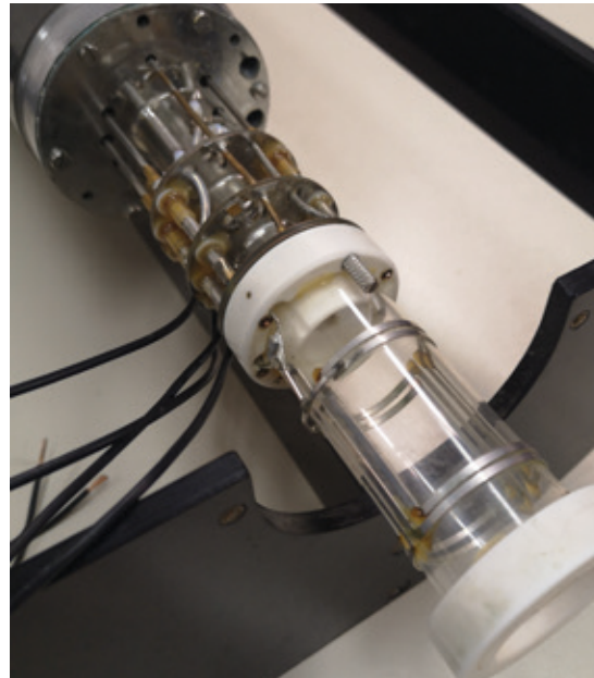
Slika 4: Primer oddajno-sprejemne RF tuljave, instalirane v RF sondu, ki se uporablja na Institutu Jožef Stefan v laboratoriju za MR slikanje.
