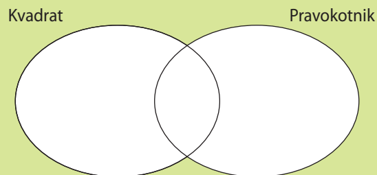
Slika 2: Vennov diagram
