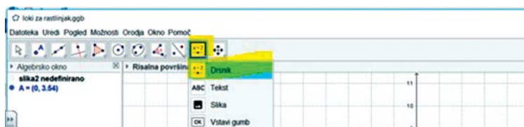
Slika 4: Izbira drsnikov
