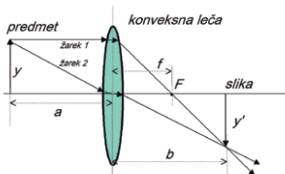
Slika 1: Konvexna leča (kot jo imamo tudi v očesu) preslika predmet v realno sliko. Razdalja b od leče do slike na mrežnici je pri očesu fiksna. Skica je smiselna tudi za oko kot celoto, če f razumemo kot skupno goriščno razdaljo vseh refraktivnih delov očesa in ne le leče kot posameznega elementa. (Vir: lastni)
