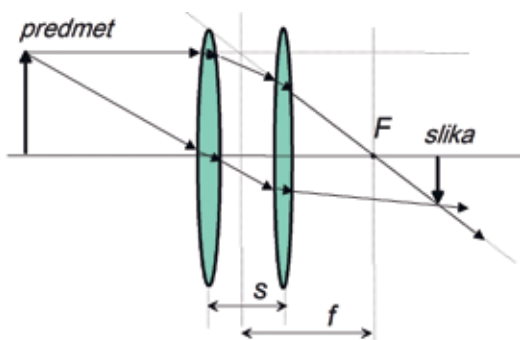
Slika 2: Dve zaporedno postavljeni leči v razdalji s upodobita predmet podobno, kot če bi uporabili eno samo, ki pa bi imela manjšo goriščno razdaljo f od obeh, kar velja, če je s dovolj majhna. (Vir: lastni)
