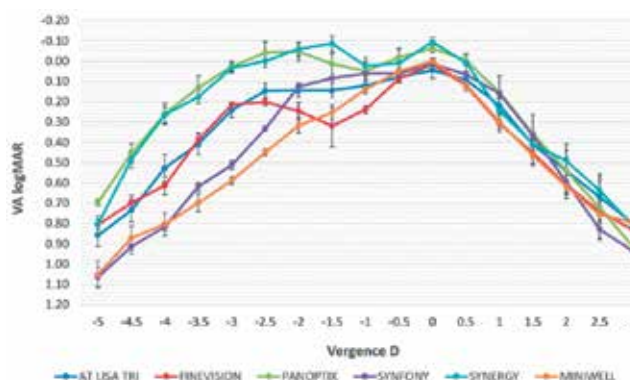
Slika 18: T. i. defokusne krivulje nekaj najbolj znanih IOL. At Lisa Tri (Carl Zeiss), FineVision (PhysIOL), Panoptix (Alcon), Symphony in Synergy (J & J) in Miniwell (SiFi). Krivulje lahko razumemo kot povezavo med neostriino v logMAR (ordinata) in razdaljo, na kateri gledamo predmet, ki je podana kot -1/D . Za pravilno vstavljeno lečo je pomemben le del od izhodišča do dioptrije 0. »Najostrejša« imajo logMAR okoli 0, zaželeno je, da v čim širšem razponu dioptrij (tj. na različnih razdaljah), krivulja pa naj nima izrazitih vrhov (npr. Symphony), ki prispevajo k občutku neostrine na vmesnih razdaljah. [14]
