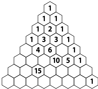
Preglednica 1: Vsota števil na lihih in sodih mestih
