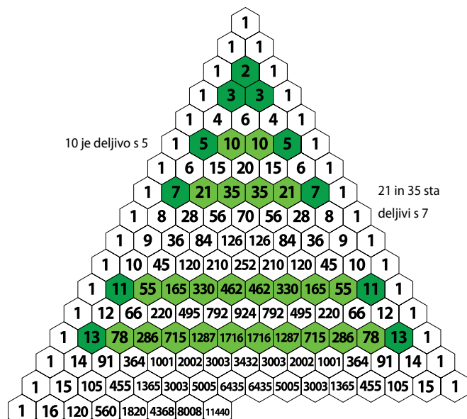
Slika 5: V vrstici, ki ima v drugem in predzadnjem polju praštevilo, so tudi vsa števila med tema dvema prašteviloma deljiva s tem praštevilom.
