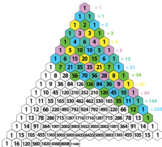
Slika 7: Vsota števil po obarvanih vrsticah tvori Fibonaccijevo zaporedje
