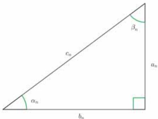
Slika 3: Pravokotni trikotnik.
