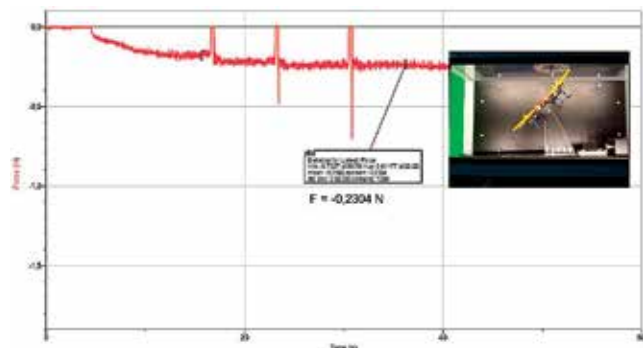
Diagram 8: F_u = 0,2304 N.
