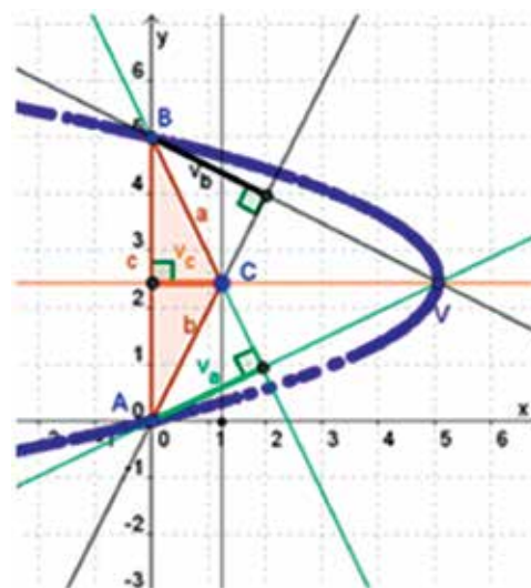
Slika 19: Geometrijsko mesto višinske točke.
