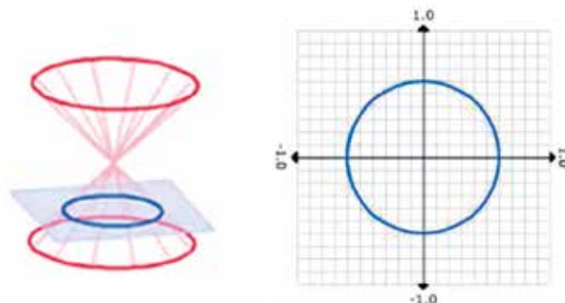
Slika 2: Presek je krožnica.
