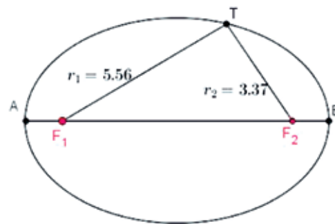
Slika 13: Geometrijska definicija elipse.
