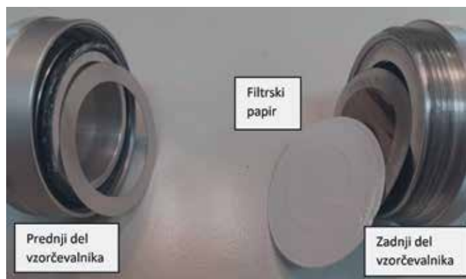
Slika 7: Vzorčevalnik je sestavljen iz dveh delov ohišja, med katera postavimo filtrski papir iz kremenovih vlaken. Področje na robu filtrskega papirja je ustrezno tesnjeno z gumijastimi in kovinskimi tesnili.
