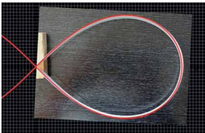
Slika 4: Primerjava oblike upognjenega traku in lemniskate.
