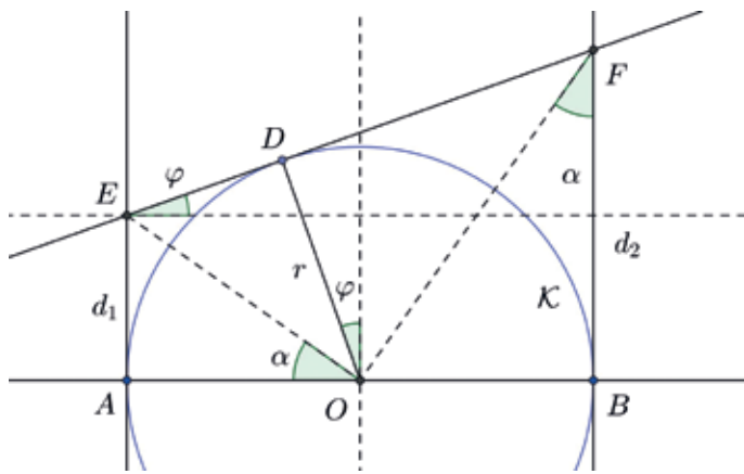
Slika 5: K dokazu enakosti d_1 d_2 = r^2 .
