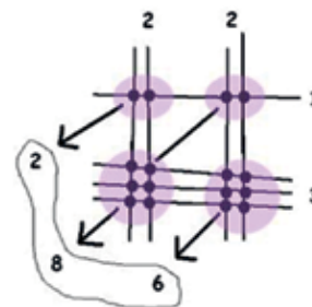
Slika 16: Grafični prikaz linijskega algoritma. (West, 2011)
