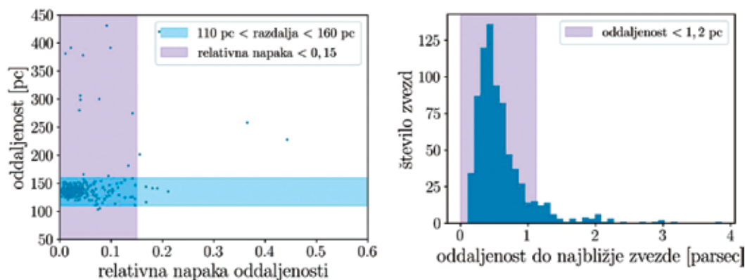
Slika 5: (Levo) Graf odvisnosti oddaljenosti zvezd od relativne napake razdalje. V preseku obarvanih pravokotnikov so zvezde, za katere predvidevamo, da so res del zvezdne kopice M45. (Desno) Histogram oddaljenosti zvezd od svoje najbližje sosedice. Zvezd zunaj obarvanega pravokotnika v naslednjem približku ne bomo upoštevali, saj so preveč oddaljene od najbližje sosedice.
