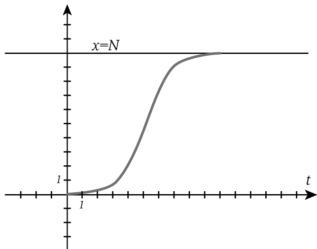
Slika 1: Logistična krivulja
