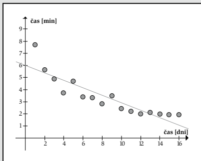
linearna funkcija
