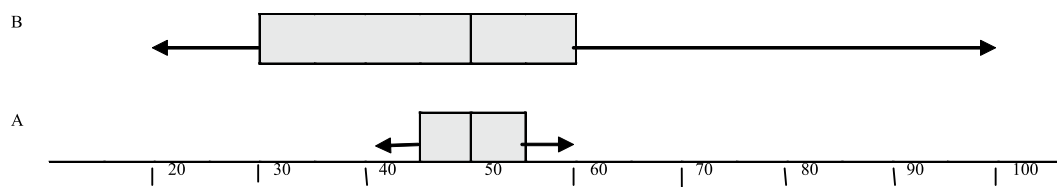
Slika 1: Prikaz hitrosti avtomobilov za Vilharjevo cesto (B) in Podpeško cesto (A) s škatlo z brki
