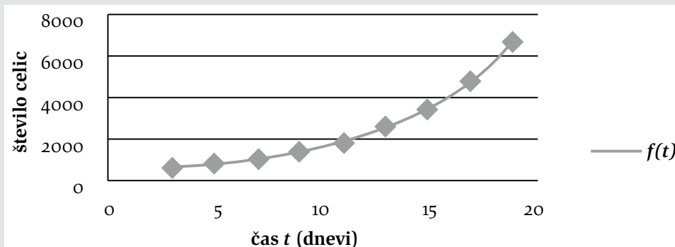
Graf: Delitev celic
