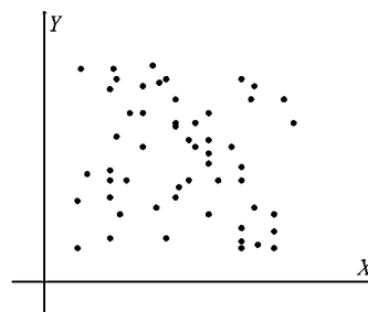
ni povezanosti
