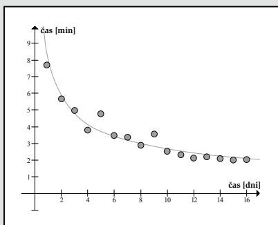
potenčna funkcija
