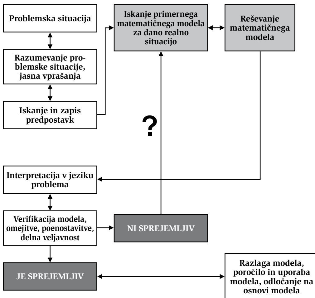
Slika 1: Proces matematičnega modeliranja
